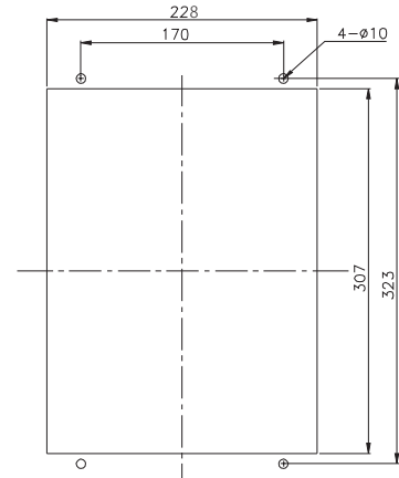
(パネルカット寸法)
