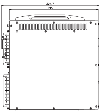
(側面図)
