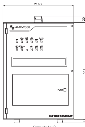
(正面図)
