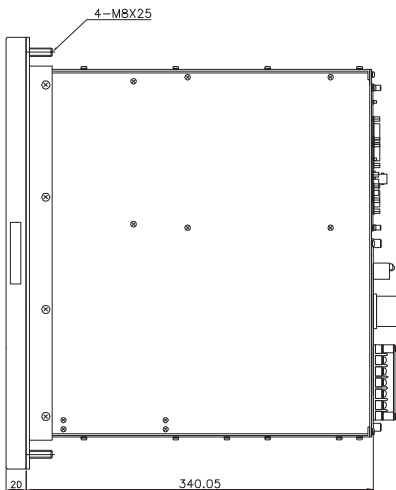
(側面図)
